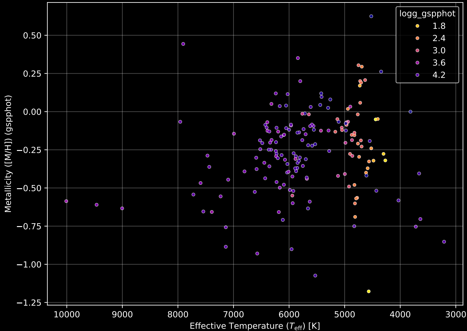
APOGEE DR17 Field: [CVZ_OB21_btx] Stellar Population Parameters (n= 175)
